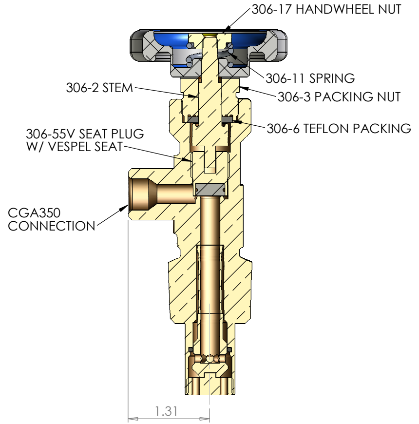
SECTION A-A SCALE 1 : 1.5
